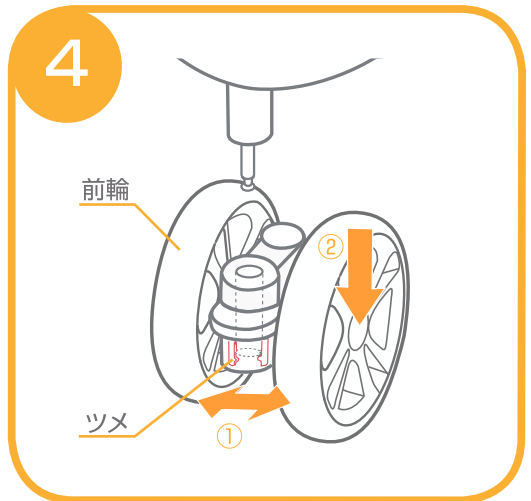
4.前輪を取り外す場合は、①前輪の内部にあるツメを開いて、②取り外して下さい。
