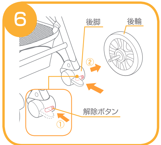
6.後輪を取り外す場合は、①後脚に付いている解除ボタンを押して、②後輪を取り外して下さい。
