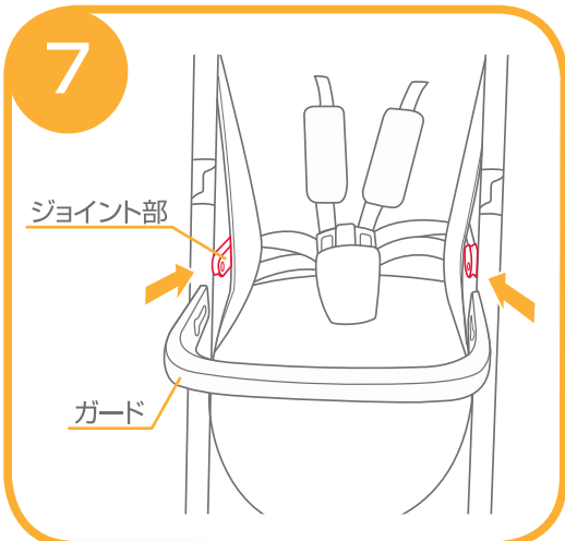
7.ガードを本体の両側に付いているジョイント部に差し込んで下さい。
