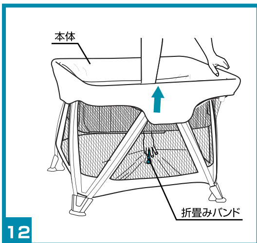
12. 本体からマットを取り外し、本体の床面に付いている折り畳みバンドを引き上げて下さい。※バスケットは付いたままでも折畳むことができます。
