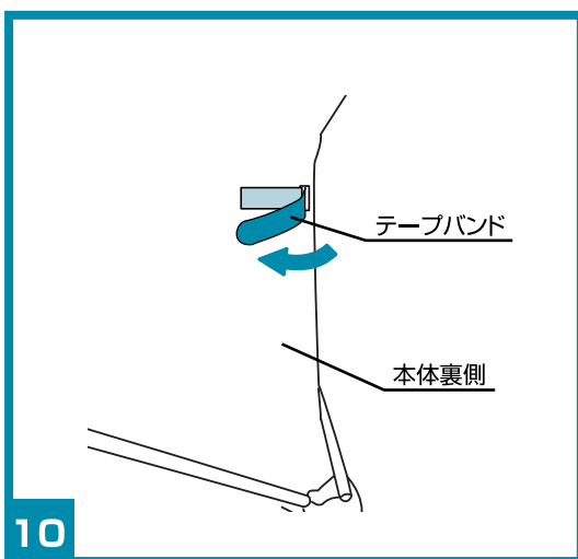
10. マットについているテープバンドを本体床面の穴に通して裏側に貼り付けて下さい。(2箇所)
