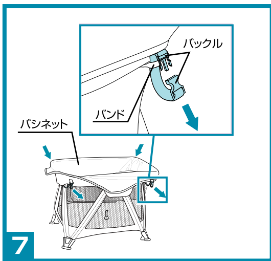
7. バスケットのバックルを外して、本体のバンドから抜き取って下さい。(4箇所)
