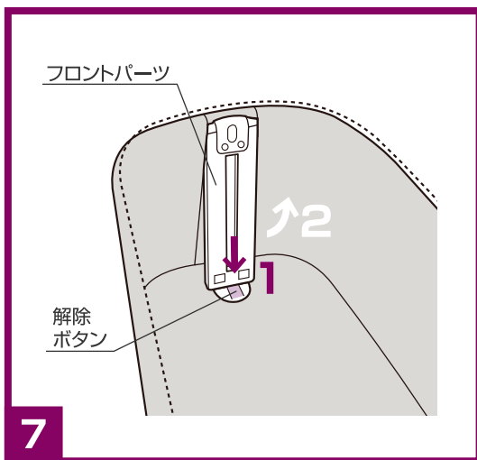
7. フロントパーツ、リアパーツを外す時は、キャリアコットの解除ボタンを押して下さい。
