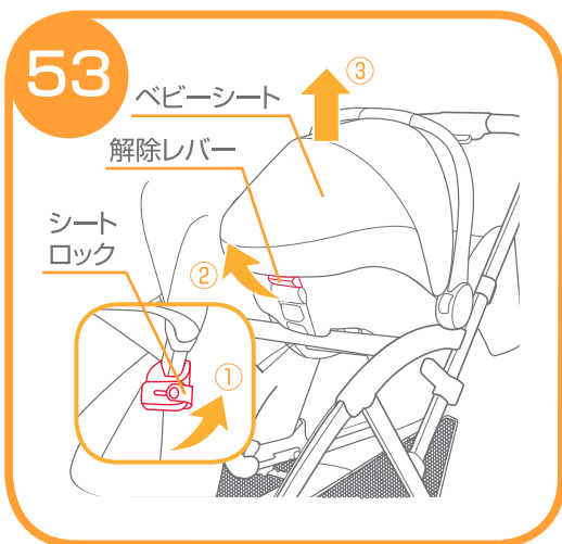
53.ベビーシートを取り外す場合は、①シートロックを引っ掛け、②ベビーシートの解除レバーを上げて、③ベビーシートを取り外して下さい。
