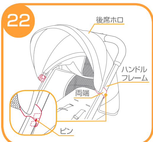
22.後席ホロの両端はハンドルフレームのピンを挟むように取り付けて下さい。
