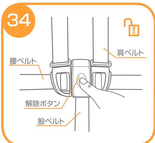
34. シートベルトを取り外す場合は、股ベルトの解除ボタンを押して、腰ベルトと肩ベルトを取り外して下さい。
