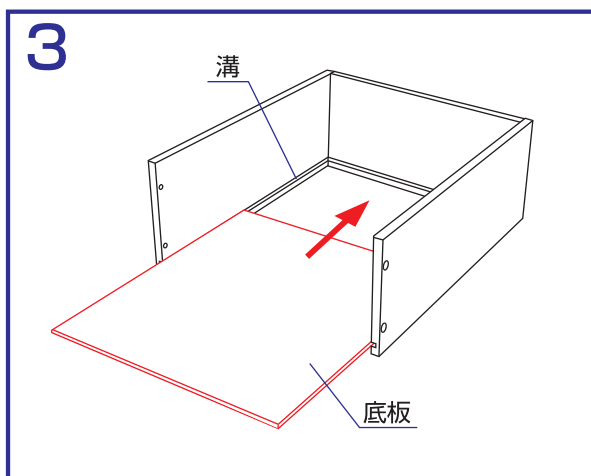
3.底板を溝に差し込んで下さい。
