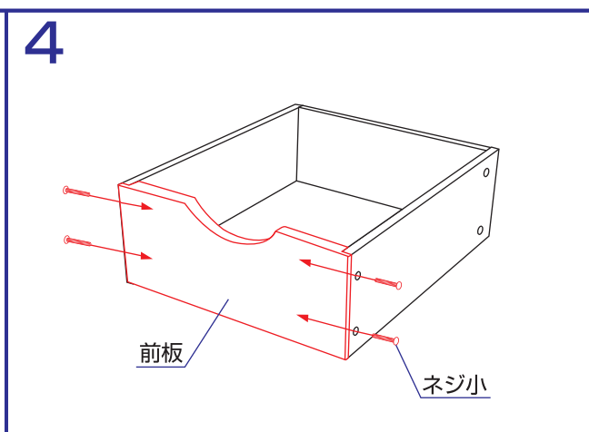
4.前板をネジ小で取り付けして下さい。※仮止めをしていた全ての箇所のネジ小を確実に締め付けて下さい。
