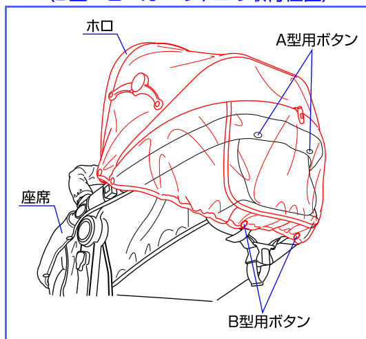
〈B型ベビーカーのホロの取付位置〉
