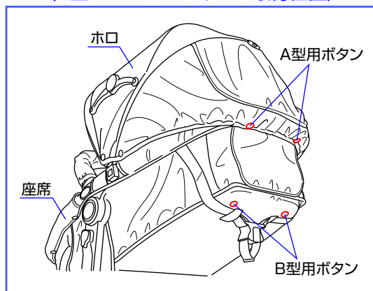
〈A型ベビーカーのホ口の取付位置〉
